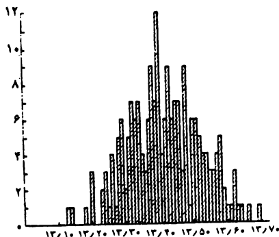
شکل ۶: نمودار پراکندگی قطر ۲۰۰ قطعه با رده‌بندی به فاصله ۰/۰۱ میلی‌متر
