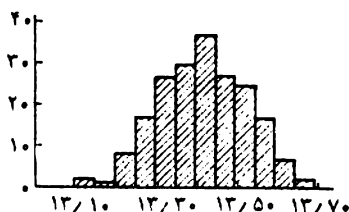
شکل ۵: جدول و نمودار پراکندگی قطر ۲۰۰ قطعه تولیدی با رده‌بندی به فاصله ۰/۰۵ میلی‌متر
